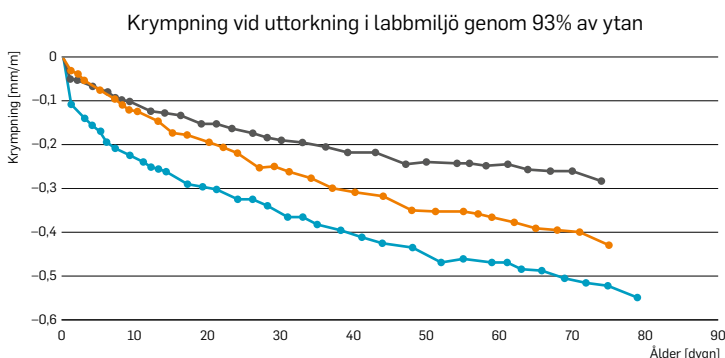
Figur 4. Krympförlopp i labbmiljö för traditionell betong (C20), lågcementbetong (LCB) och cementbunden makadam (CBM). Den relativa fuktigheten i labbet sjönk successivt från 60 till under 30 procent.
