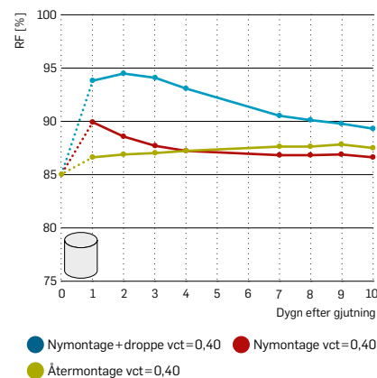
Efter knappt två veckor når de uppfuktade hålen samma nivå som övriga i hinken. Hinkarna har stått med lock sedan gjutning och är 18 månader gamla. Betongen är gjuten med gamla Bascement.
