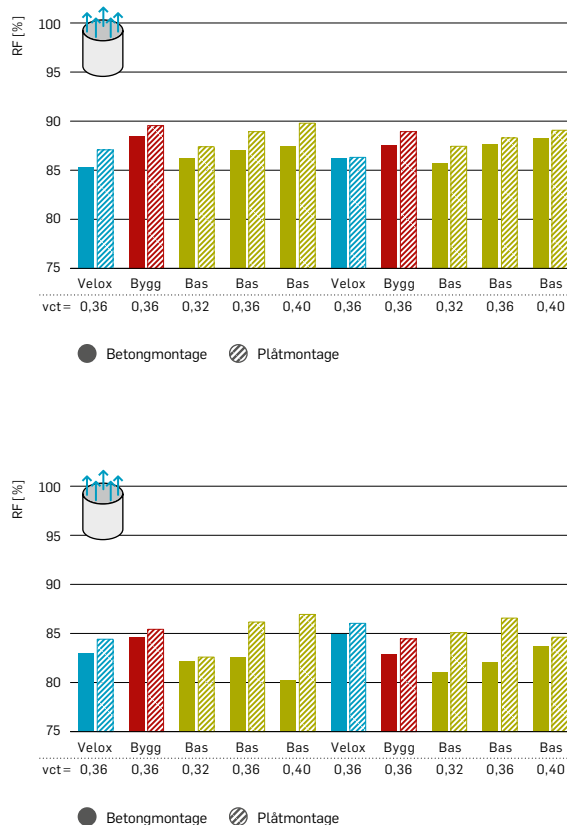
Figur 2. Betong vs. Plåtmontage. Betonghinkar som stått med öppet lock inomhus i 20 grader. Varje hink har två HumiGuard-givare. Den första har monterats ovanifrån och tätats mot betong medan den andra monterats från sidan och tätats mot plåt. Båda givarna sitter på ekvivalent mät djup räknat från betongytan. Vid montaget och avläsning av givarna är betongen drygt 2 månader gammal. Höjden på betongen är ca 17 cm. (Slite Velox CEM I, Skövde Byggcement CEM II/A-LL, Slite Bascement CEM II/A-V)
