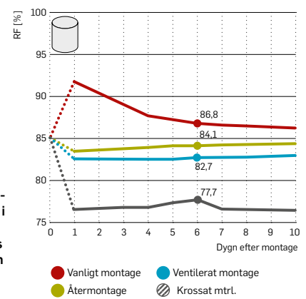
Figur 5b. RF-utvecklingen för tre olika varianter på en borrhålmätning samt ett uttaget prov för en betong med Basement. Hinkarna hade stått med lock i ett år vid provningstillfället. Från första montage av HumiGuard-givare tills hinken spräcks går det ca 4 veckor och därefter ytterligare två dygn innan en ny givare monteras i provröret.
