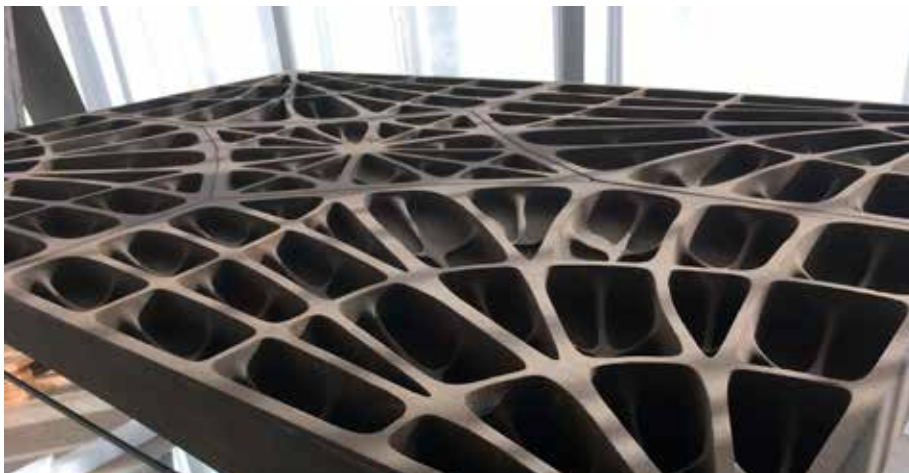
3D-printing av dubbelkrökta betongstrukturer. Roboten skapar först önskad topologisk form på grusbädden och printar sedan betong ovanpå. [RobArch 2018, ETH Zürich].
